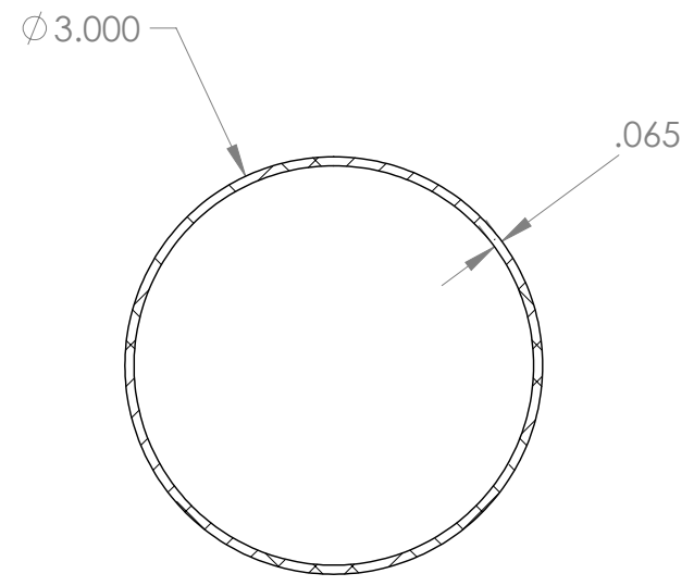
SECTION A-A SCALE 1 : 1.5
